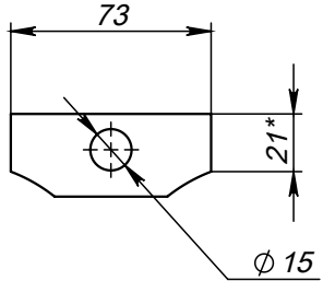
Поз.4 (Ушко) развертка
