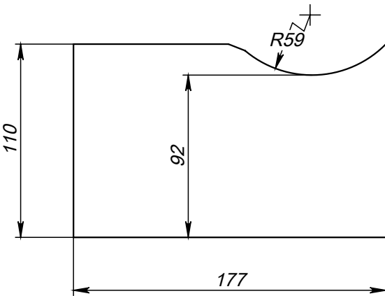
Поз.2 (Угольник) развертка
