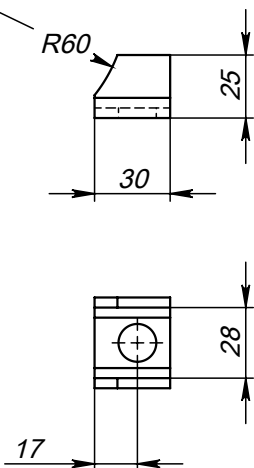
Поз.4 (Ушко)
