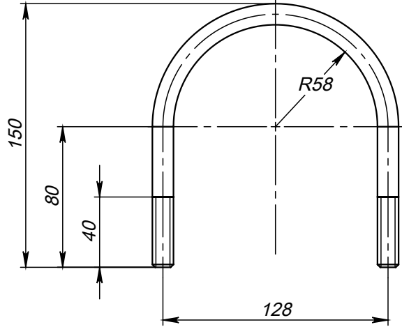
Поз.5 (Хомут)
